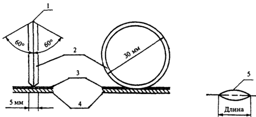
Рисунок 18 - Прибор для вдавливания
