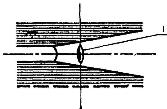
Рисунок 20 - Расположение источника света и микроскопа
